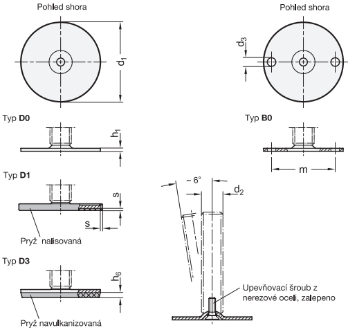
Provedení se závitovým čepem
