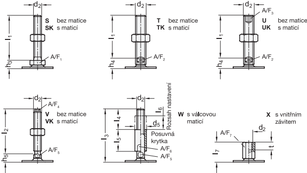
Provedení se závitovým čepem
